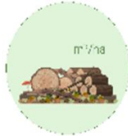
Totholz (liegend)
